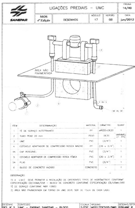
FIGURA 2.147 - MODELO DE INSTALAÇÃO DE CAVALETE. FONTE: SANEPAR, 2012.
