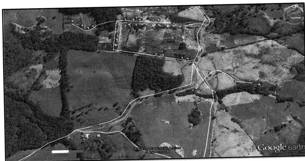
FIGURA 2.171 – LOCALIZAÇÃO DO RESERVATÓRIO EM RELAÇÃO À CAPTAÇÃO DA VILA RURAL BARRA BONITA. FONTE: GOOGLE EARTH (2014), ORGANIZADO POR AMBIENTAL COSTA OESTE.
