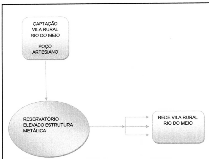
FIGURA 2.189 – FLUXOGRAMA DO SISTEMA DE ABASTECIMENTO DA VILA RURAL RIO DO MEIO.
