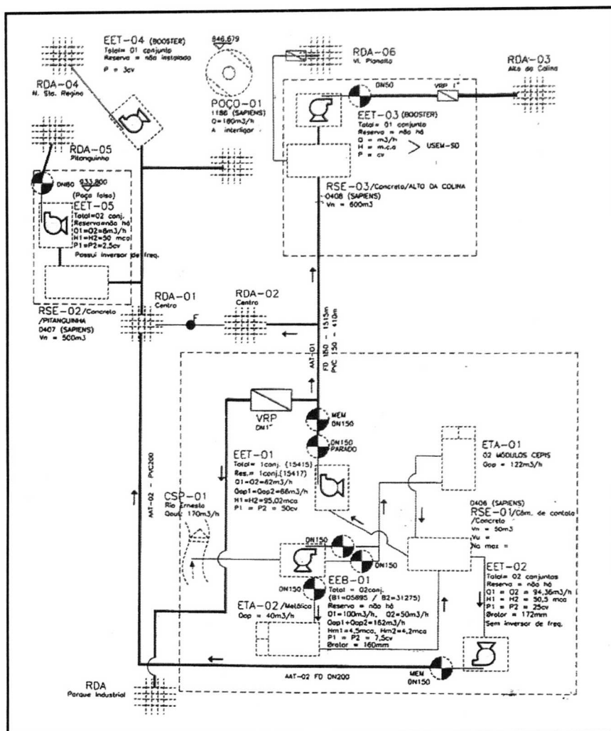
FIGURA 2.148 – FLUXOGRAMA DE ABASTECIMENTO DE ÁGUA DE PITANGA – PR. FONTE: SANEPAR, 2015.
