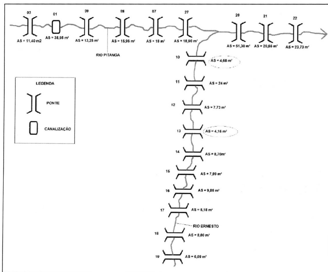
FIGURA 2.267 – ESQUEMA DE PONTES E CANALIZAÇÕES DOS RIOS ERNESTO E PITANGA. FONTE: AMBIENTAL COSTA OESTE (2015).
