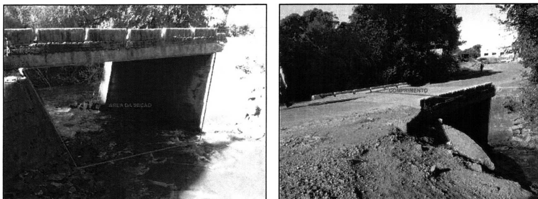
FIGURA 2.240 – VISTA DO PONTO 03 COM AS DEFINIÇÕES DE “ÁREA DA SEÇÃO” E COMPRIMENTO.
