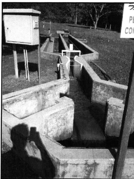
FIGURA 2.220 – CALHA PARSHALL ETE PITANGA. FONTE: TRABALHO DE CAMPO, AMBIENTAL COSTA OESTE (2014).
