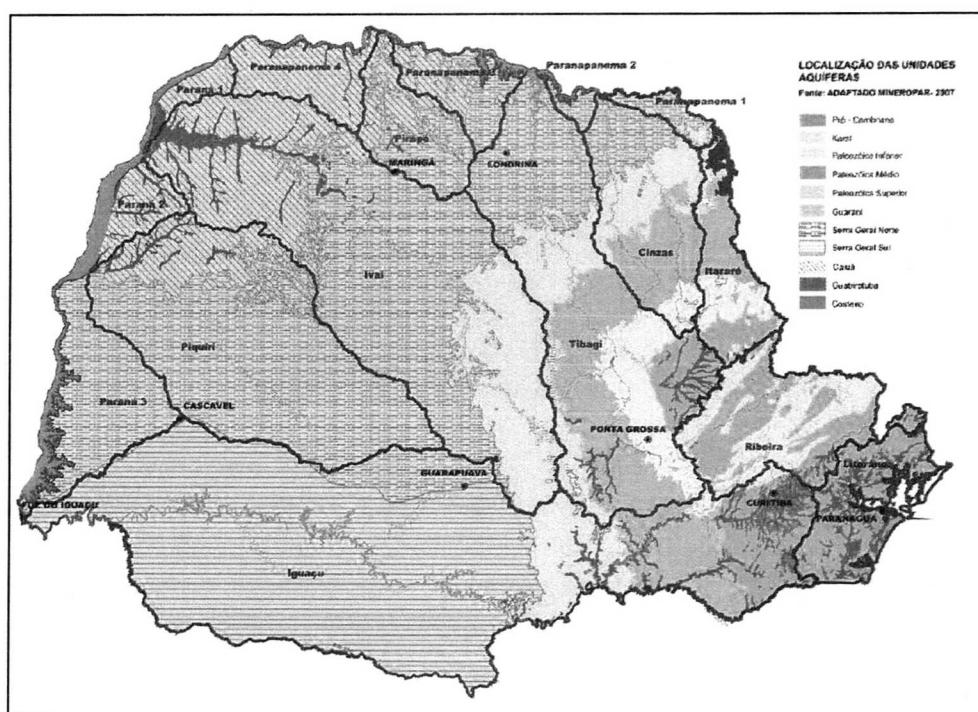
FIGURA 2.150 - UNIDADES AQUÍFERAS DO ESTADO DO PARANÁ FONTE: SEMA PR (2010).
