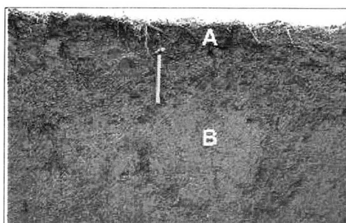
FIGURA 2.40 – PERFIL DE NITOSSOLO FOTO: OROMAR JOÃO BERTOL
