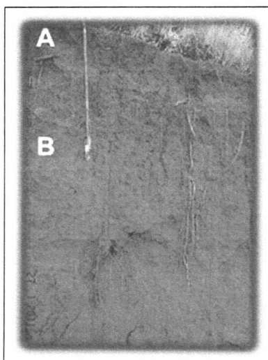
FIGURA 2.36 – PERFIL DE LATOSSOLO. FOTO: MARCELO RICARDO DE LIMA
