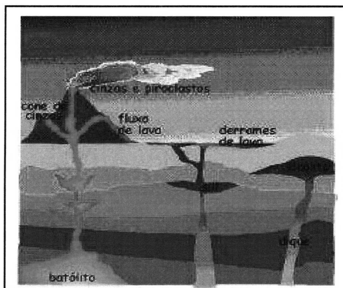
FIGURA 2.34 – ESQUEMÁTICAS A FORMAÇÃO DE ROCHAS ÍGNEAS. FONTE: WWW.SCIELO.BR (2005)
