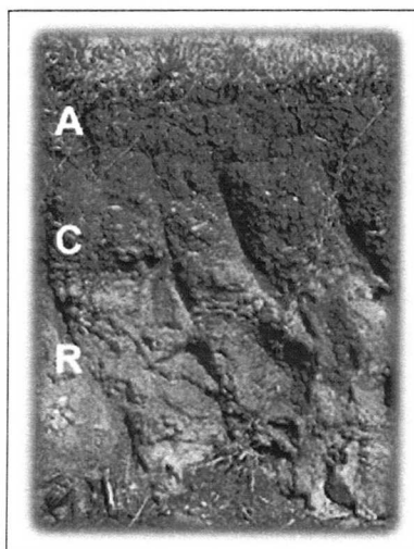
FIGURA 2.38 – PERFIL DE NEOSSOLO FOTO: MARCELO RICARDO DE LIMA
