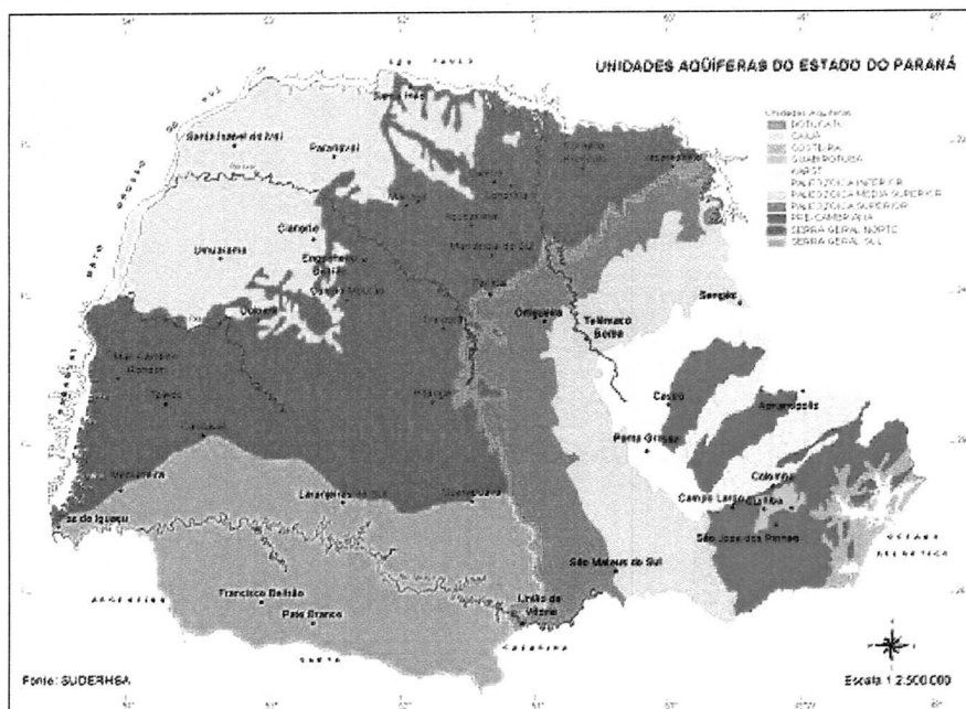
FIGURA 2.45 – UNIDADES AQUÍFERAS DO PARANÁ FONTE: SUDERHSA
