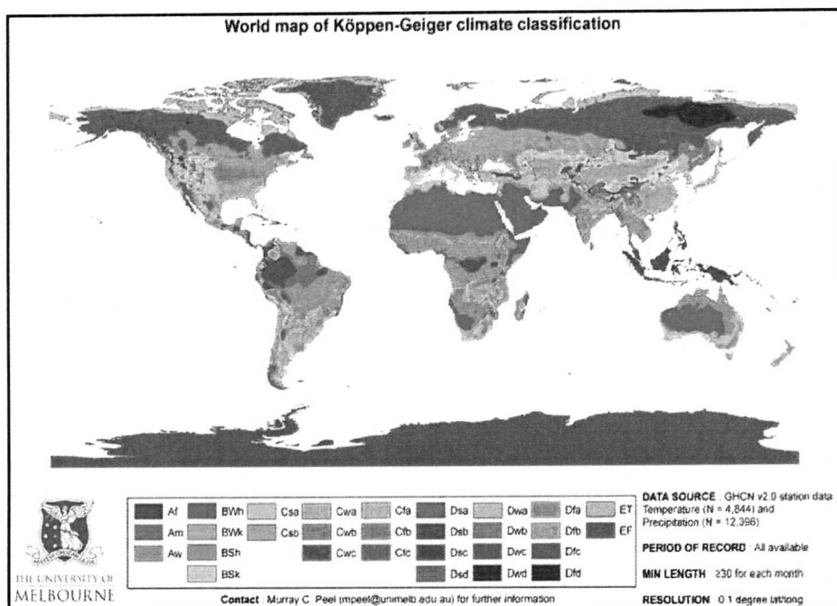
FIGURA 2.32 – MAPA DA CLASSIFICAÇÃO CLIMÁTICA DE KÖPPEN FONTE: HTTP://PT.WIKIPEDIA.ORG/WIKI/FICHEIRO:WORLD KOPPEN MAP.PNG
