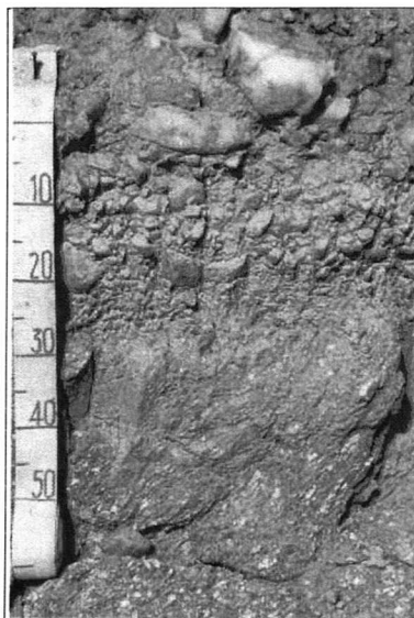
FIGURA 2.41 – NEOSSOLOLÍTOLICO FONTE: EMBRAPA
