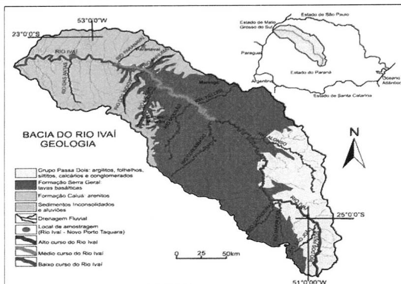
FIGURA 2.33 – GEOLOGIA DA BACIA DO IVAÍ FONTE: OUTRAGEOGRAFIA.BLOGSPOT.COM.BR/2013
