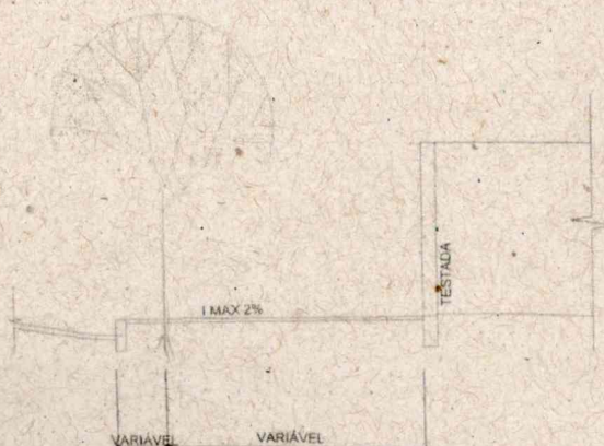
CORTE 1 ESCALA 1/75
